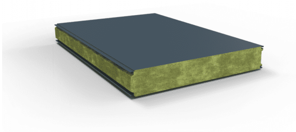
Rysunek 4.2: Płyta ścienna GS MW CH
